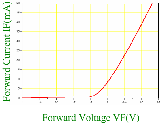
IF-VF(Ta=25°C)
